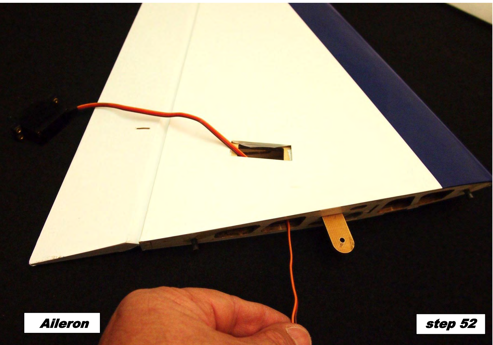
Aileron
